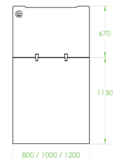
Cloison semi-vitrée
