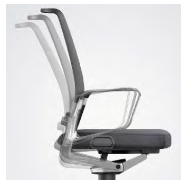
Smart Motion Technology : inclinaison automatique du coussin d'assise. Tension du dossier réglable individuellement. Mouvement additionnel du bassin. Favorise la stimulation accrue de la musculature du torse, l'assise est plus dynamique et bénéfique pour la santé.
