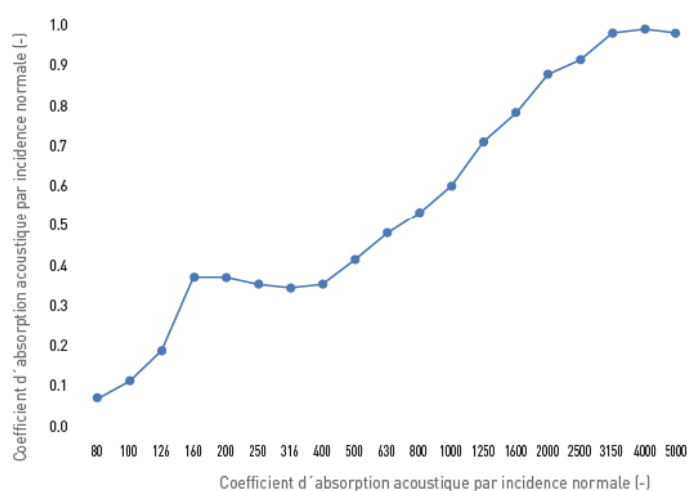
Coefficient d'absorption acoustique - UNE EN ISO 354:2004
