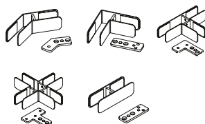
Pièces de liaison Pour cloisons pieds plats Finition Blanc (WT), Alu. (WA) ou Noir (BL)
