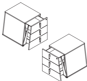
Caissons mobiles inclinés 3 tiroirs L43/51 x P57 x H57 cm Tiroirs internes en métal Avec compartiment privatif
