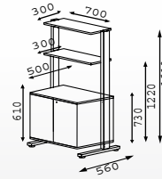
Armoire basse avec 2 tablettes rehausse
