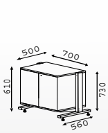
Armoire basse et roulettes
